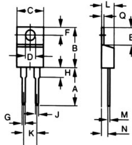
Dimensions TO-220AC
