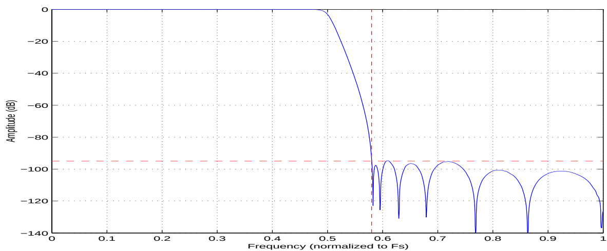
Figure 22. SSM Stopband
