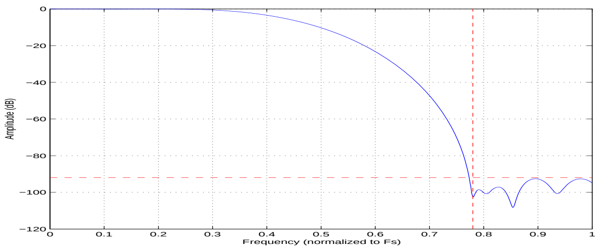
Figure 24. QSM Stopband
