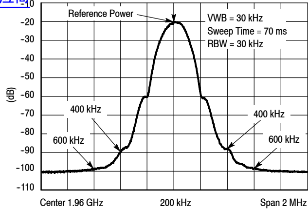
Figure 11. EDGE Spectrum
