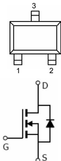
SOT-23-3
