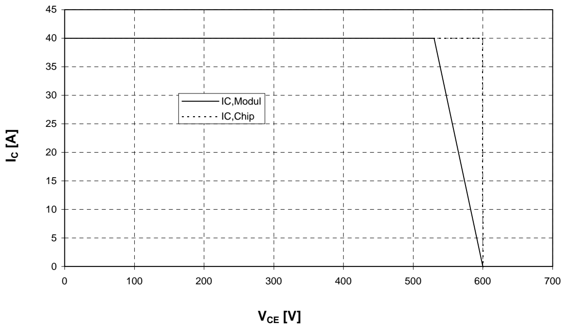
Sicherer Arbeitsbereich Wechselr. (RBSOA) I_c = f(V_{CE}) Reverse bias safe operating area Inverter (RBSOA) T_{vj} = 125^\circ\text{C}, V_{GE} = \pm 15\text{V}, R_G = 47 \text{ Ohm}
