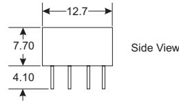
CTDD1210DF-TU1K-1 Package
