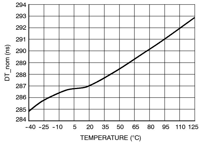
Figure 26. T_dead_nom
