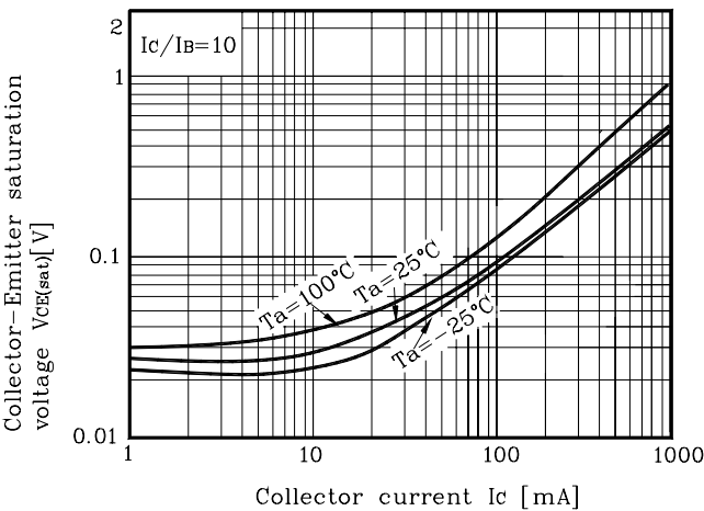
Fig. 4 V_{CE(SAT)} - I_c
