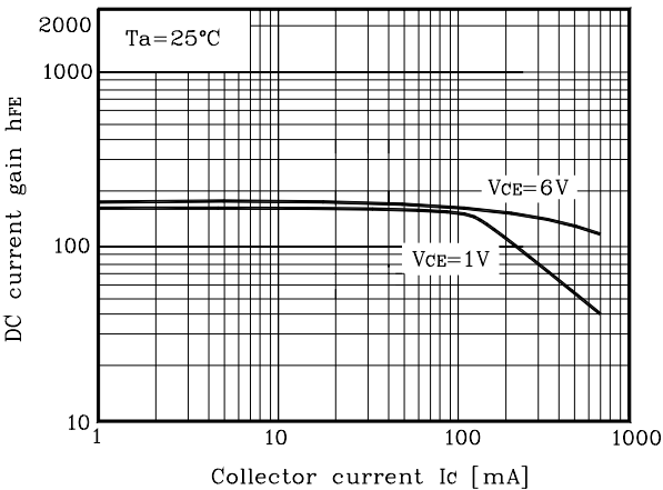
Fig. 5 h_{FE} - I_c
