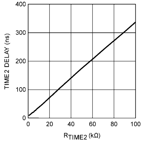
Time2 Delay vs R_{TIME2} (k \Omega )
