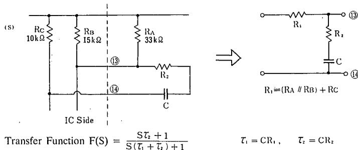
Fig. 3 NJM2206 LPF
