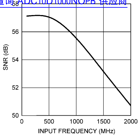
SNR vs. INPUT FREQUENCY (ADC10D1000) 查询"ADC10D1000NOPB"供应商
