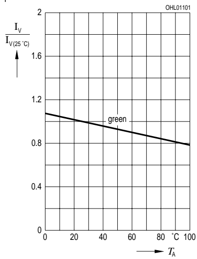
Relative Lichtstärke I_V / I_{V(25\text{ °C})} = f(T_A)
