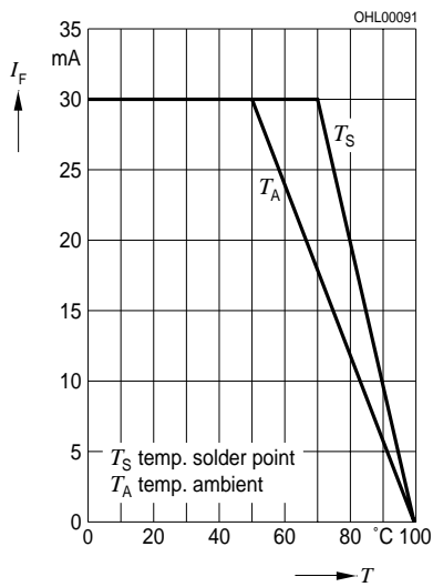
Maximal zulässiger Durchlassstrom I_F = f(T_A)
