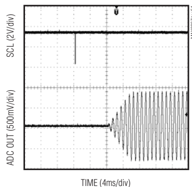
ADC SOFT-START
