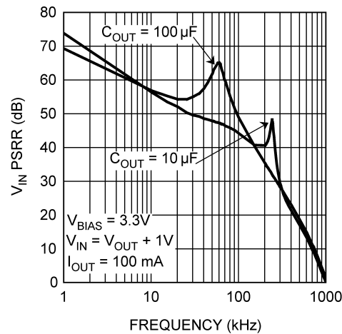
V_{IN} PSRR
