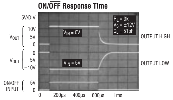
LT1032 • TPC13
