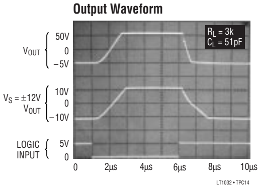
LT1032 • TPC14
