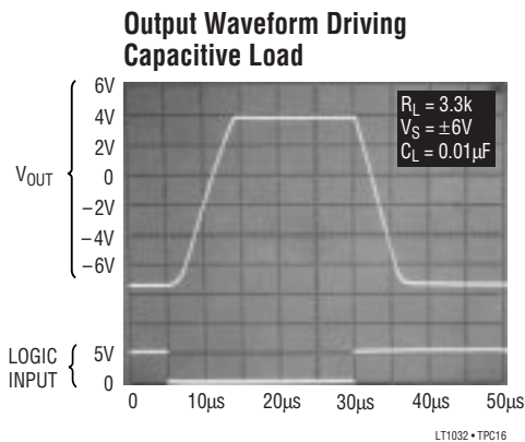
LT1032 • TPC16
