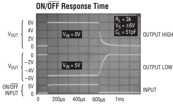
LT1032 • TPC12
