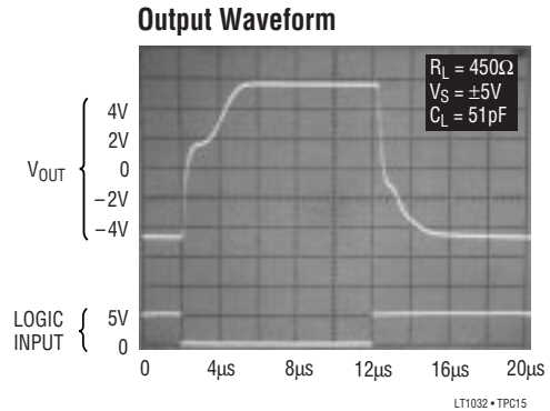
LT1032 • TPC15
