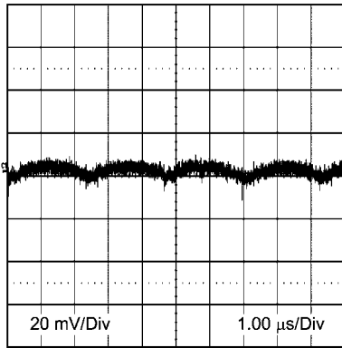
Output Ripple 24V_{IN} 3.3V_O 2A, BW = 200 MHz
