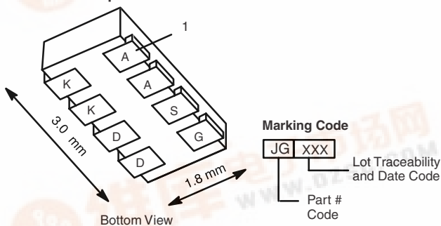
1206-8 ChipFET®
