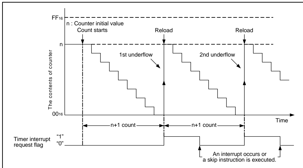
Fig 30. Auto-reload function
