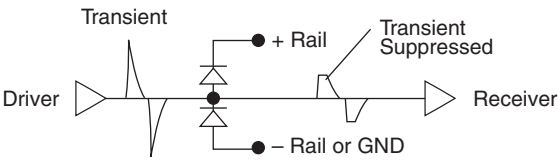
ESD Suppression
