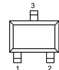
SOT-23-3
