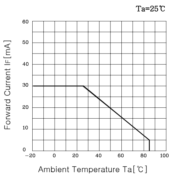
Fig. 3 I_F - T_a
