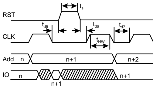
图6 写操作时序
