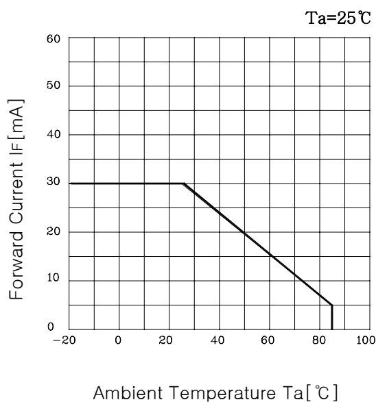
Fig. 3 I_F - T_a
