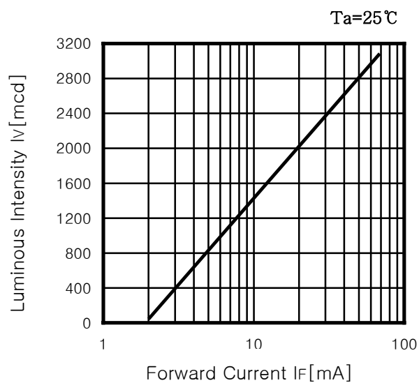
Fig. 2 I_V - I_F
