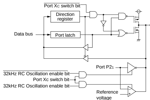
(10) Port P20
