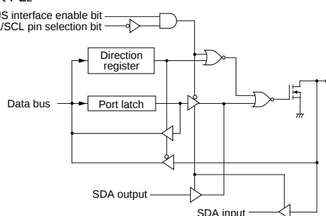
(12) Port P22
