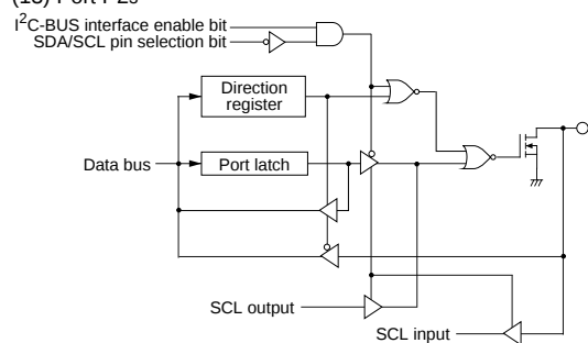
(13) Port P23
