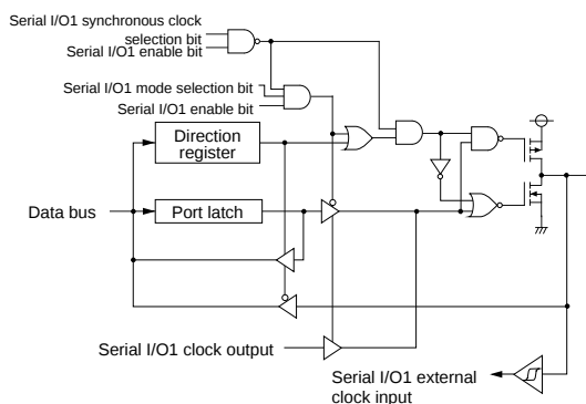
(16) Port P26
