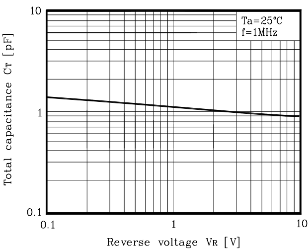
Fig. 2 C_T - V_R
