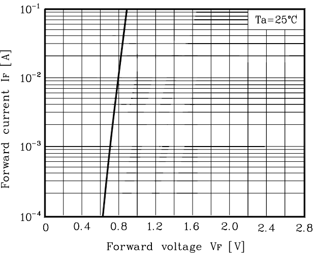
Fig. 3 I_F - V_F
