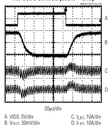
DYNAMIC VID CODE CHANGE (D0 = 12.5mV)
