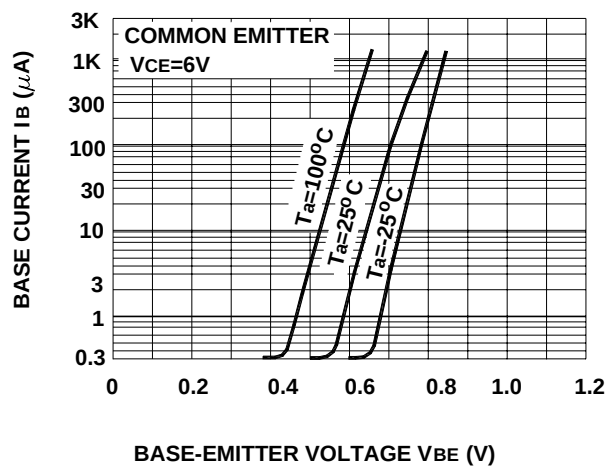
I_B - V_{BE}
