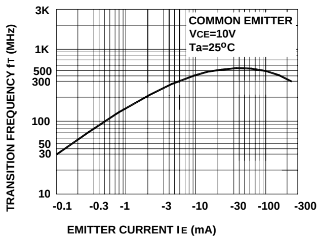
f_T - I_E
