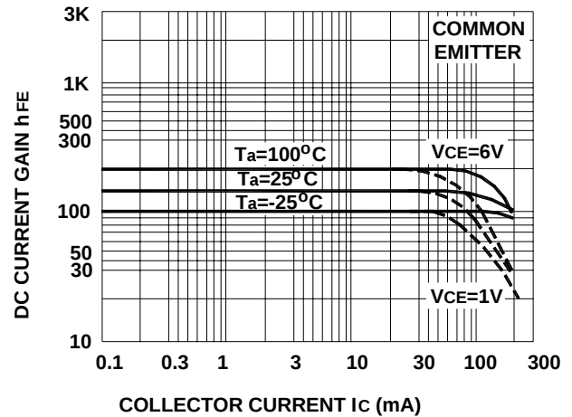
h_{FE} - I_C
