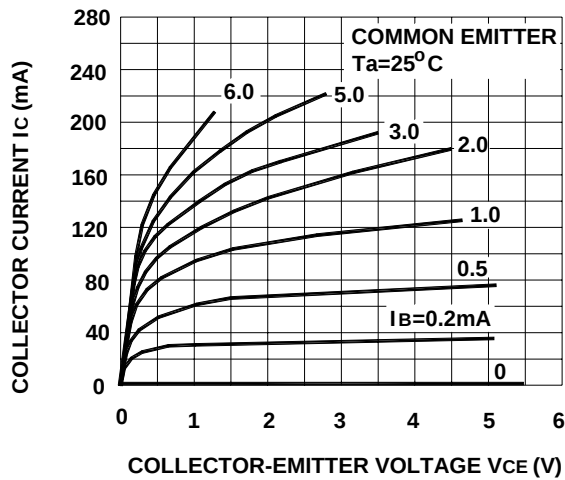
I_C - V_{CE}
