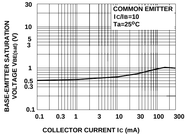
V_{BE(sat)} - I_C
