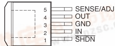
KTTP PACKAGE (TOP VIEW)
