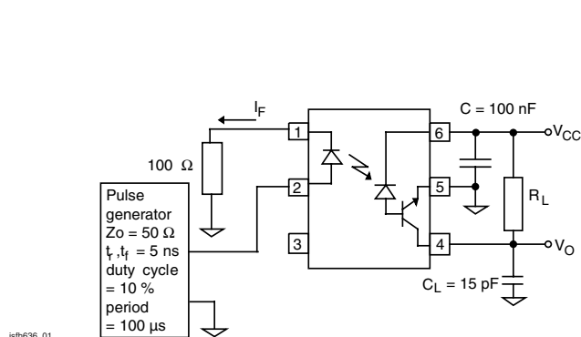
Fig. 1 - Test Setup
