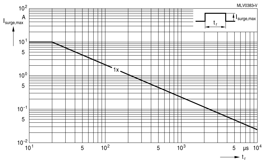
CT0402L14UG
