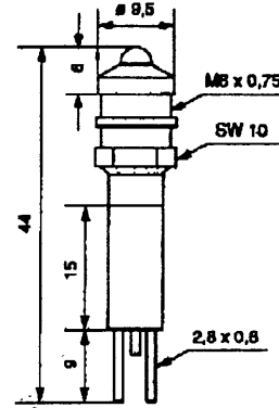
LED Signalleuchte mit Außenreflektor LED Indicator with exterior reflector
