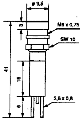
LED Signalleuchte mit Innenreflektor LED Indicator with interior reflector
