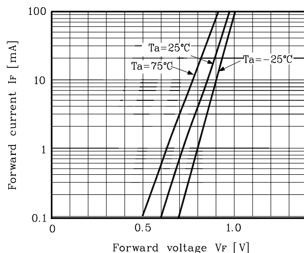
Fig. 2 I_F-V_F
