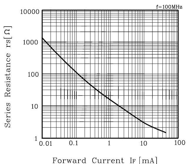
Fig. 4 r_s-I_F
