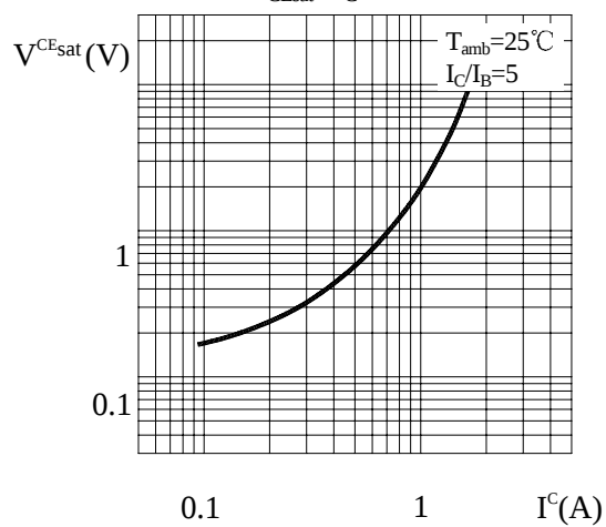
V_{CEsat} - I_C 关系曲线
