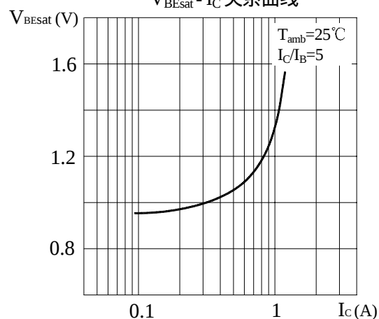
V_{BEsat} - I_C 关系曲线
