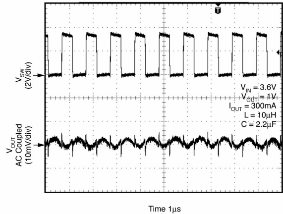
Ripple
