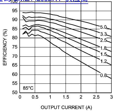
Efficiency 8V input 85°C 查询"LMZ14203EXT"供应商
