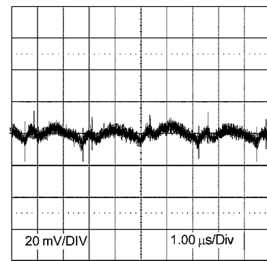
Output Ripple 24V_{IN} 3.3V_O 3A, BW = 200 MHz
