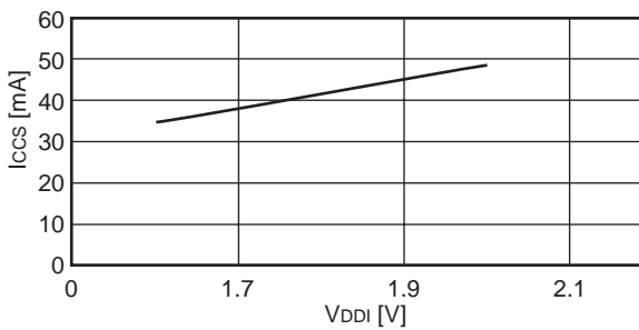
I CCS -V DD1 example characteristics Ta = +25 °C
