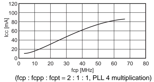
I CC -f CP example characteristics Ta = +25 °C, V DD1 = 3.3 V V DD1 = 1.8 V
