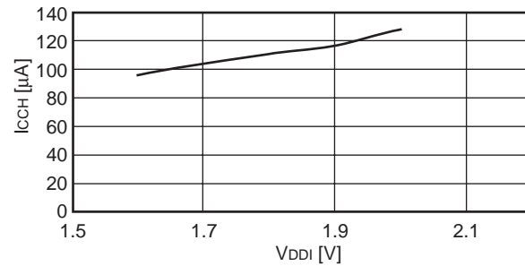
I CC H-V DD1 example characteristics Ta = +25 °C
