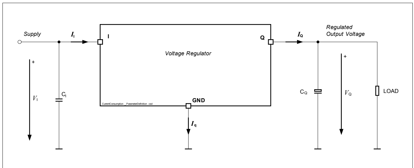
Figure 6 Parameter Definition
