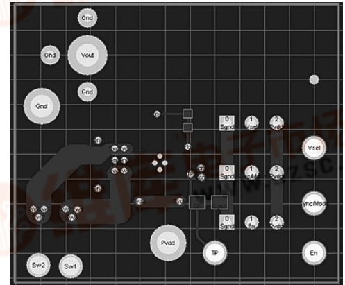
Bottom Layer
