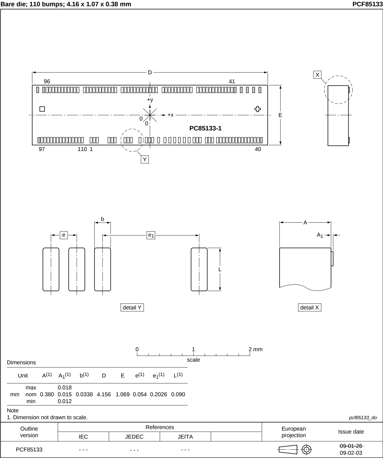
Fig 23. Bare die outline of PCF85133
