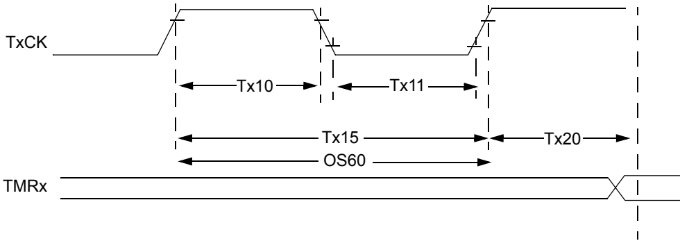
FIGURE 28-5: 64GP202 供应用
