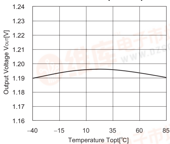
R1180x121x ( V_{IN}=2.2V )
