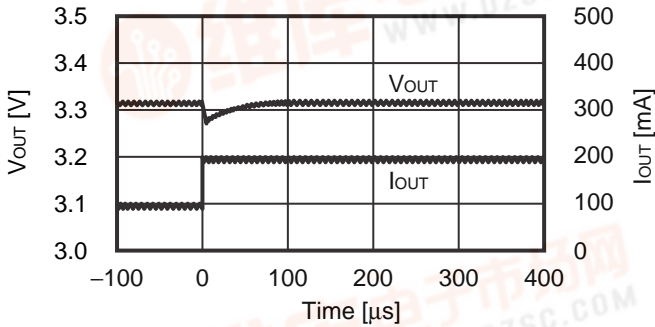
(1) I_{OUT} = 100\text{ mA} \rightarrow 200\text{ mA}
