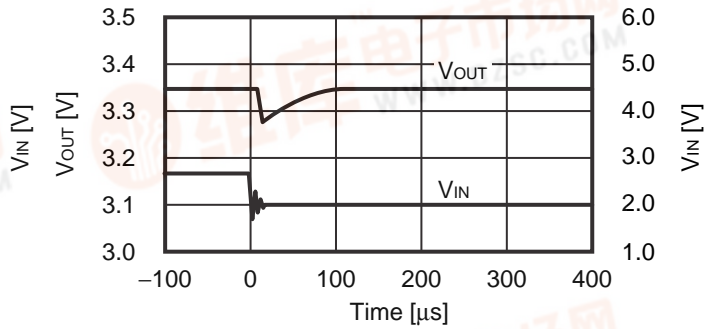
(2) V_{IN} = 2.64\text{ V} \rightarrow 1.98\text{ V}
