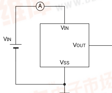
●Circuit ④
