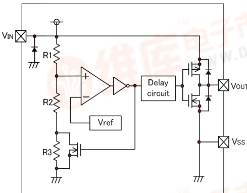
(1) CMOS output
