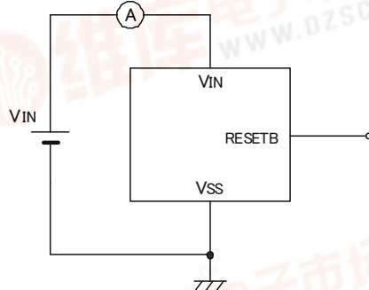
●Circuit ④
