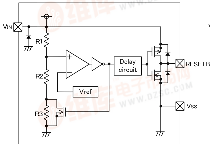
(1) CMOS output
