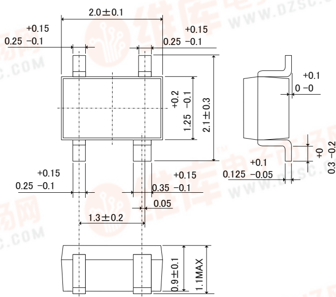
SSOT-24
