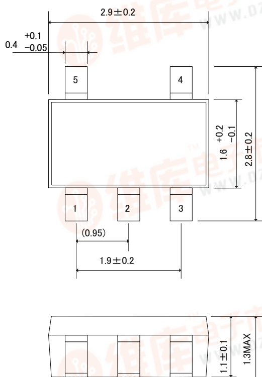
SOT-25
