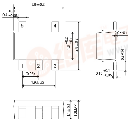
SOT-25 Package
