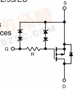
P-Channel MOSFET
