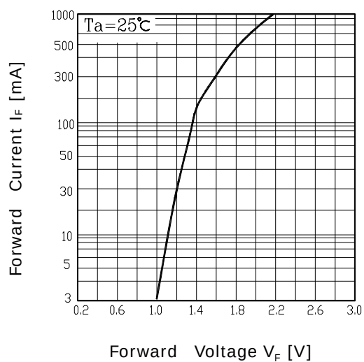
Fig. 1 I_F - V_F
