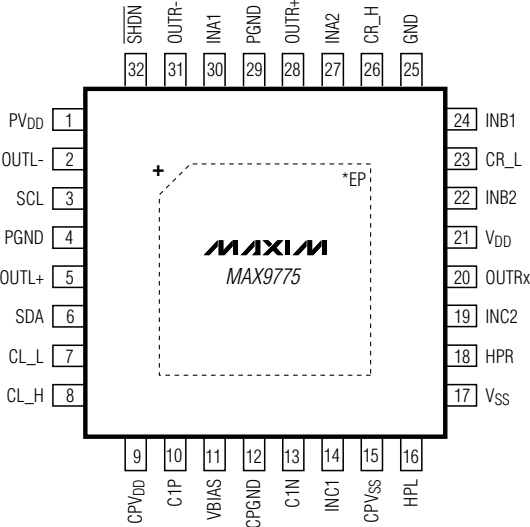
32 TQFN-EP*
